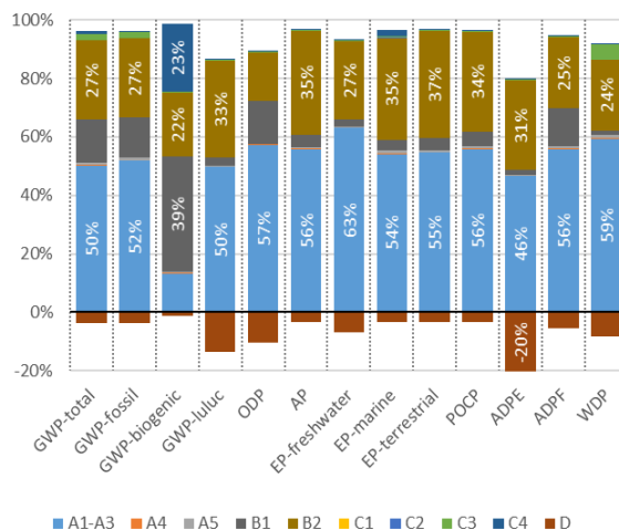
Fig. 6-2: Indicadores que describen los impactos ambientales, distribución por módulo
