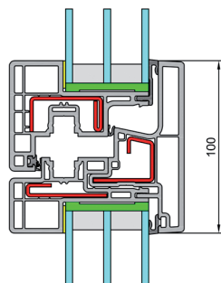
Presjek štulp/prečka
