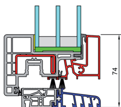
Presjek balkonska vrata sa pragom
