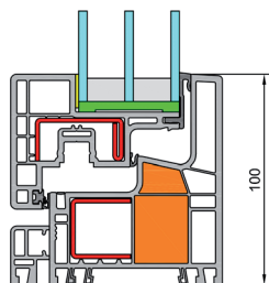
Osnovni presjek GEALAN-KUBUS®
