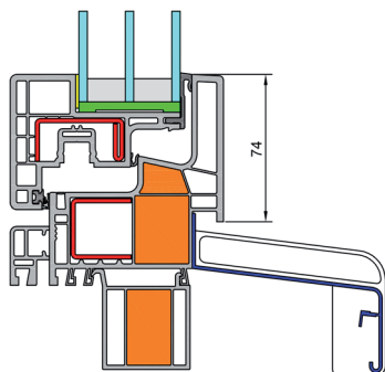
Presjek donjeg dijela
