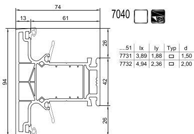
Pfosten 94 mm
