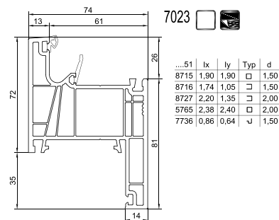
Sanierungsrahmen 72 mm
