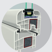
6-камерна система напівутплнена стулка
