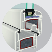
5-ти камерна система стулка зі зміщенням
