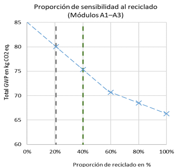
Fig. 6-1: GWP total del módulo (A1-A3) de fabricación de ventanas según contenido reciclado
